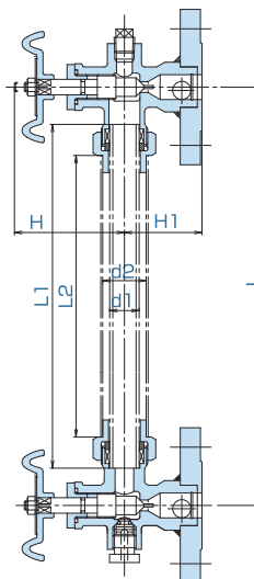
■ 10GVF-BP-14 ボールチャッキ付 プラグ弁付
